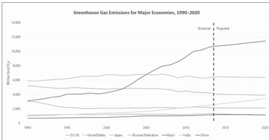
2. ábra. Az Európai unió (EU), az USA, Japán, Oroszország, Brazília, India és Kína szén-dioxid kibocsátása 1990-től napjainkig millió tonna/év egységeiben kifejezve.
