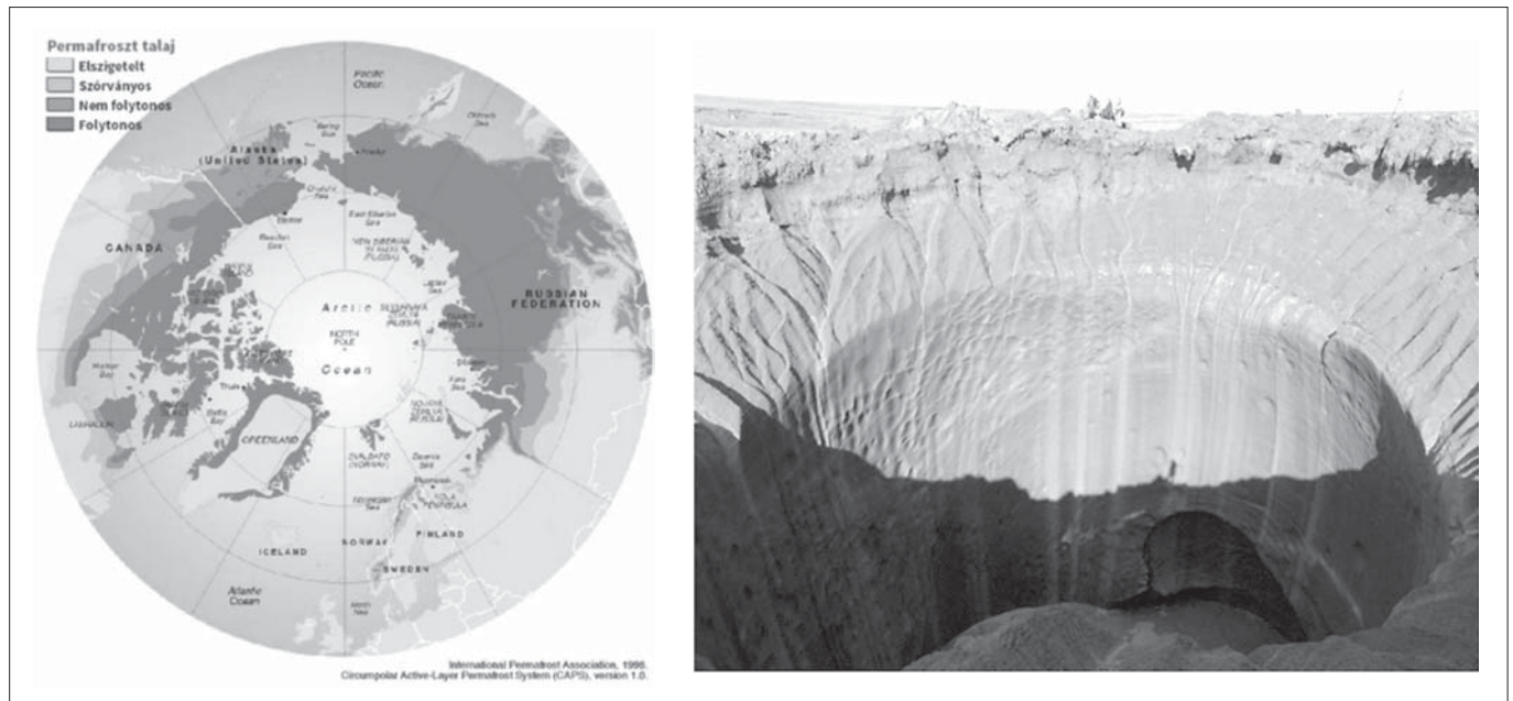
8. ábra. A jelenkori permafroszt területe és egy metánrobbanás okozta kráter a tundrán.
