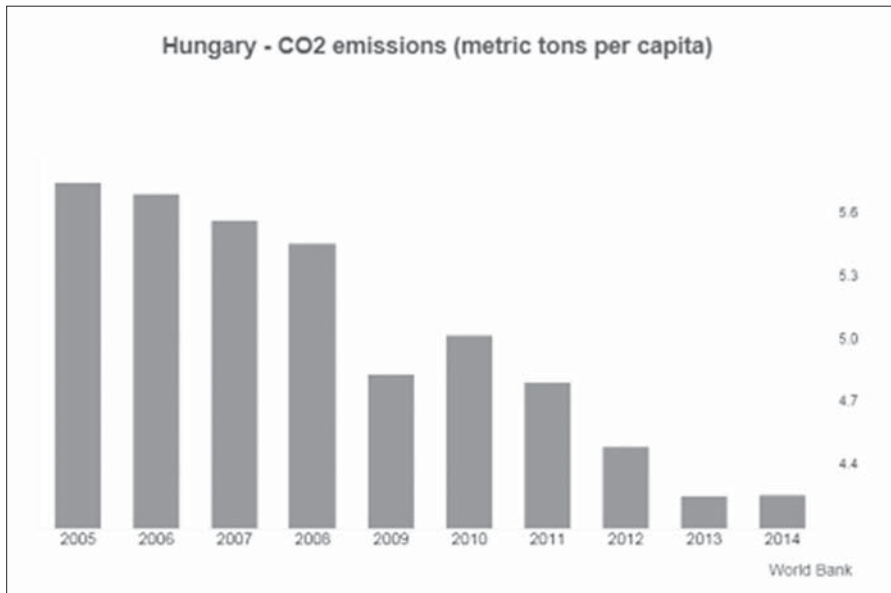
3. ábra. Az egy főre eső CO 2 kibocsátás Magyarországon 2005 és 2014 között (tonna/fő).
