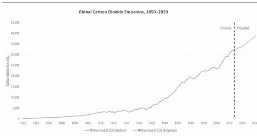
1. ábra. Az évente globálisan kibocsátott CO 2 millió tonnában kifejezve 1850-től kezdve, 2015-és 2030 között becsült érték.
