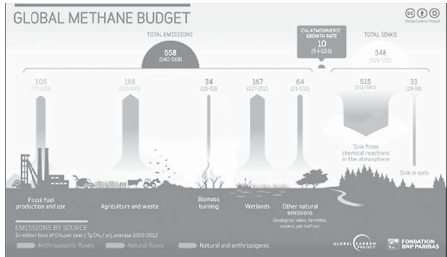
6. ábra. A globális metán-háztartás. (The Global Methane Budget 2000-2017. http://publications.jrc.ec.europa.eu/repository/handle/JRC102625 )
