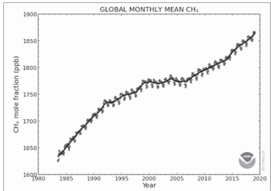
7. ábra. A metán koncentráció emelkedése ppb (part per milliárd) egységekben kifejezve az évek függvényében.
