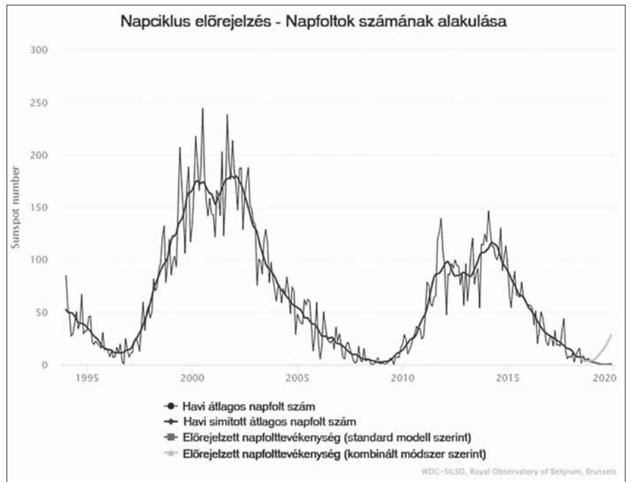
11. ábra. A napciklus alakulása jelenleg.
