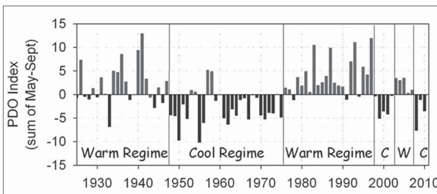
9. ábra. A Csendes-óceán évtizedenkénti hőmérséklet oszcillációja (északi szélesség 20°N fölött). A május-szeptemberi hőmérséklet-változásokat évtizedenként összegezték (Pacific Decadal Oscillation, PDO) 1925 és 2010 között.
