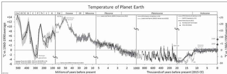
1. ábra. Hőmérsékletváltozások 500 millió évre visszamenőleg az 1960-1990-es évek közötti 30 év átlaghőmérsékletéhez viszonyítva Forrás: https://hu.wikipedia.org/wiki/%C3%89ghajlat#Data
