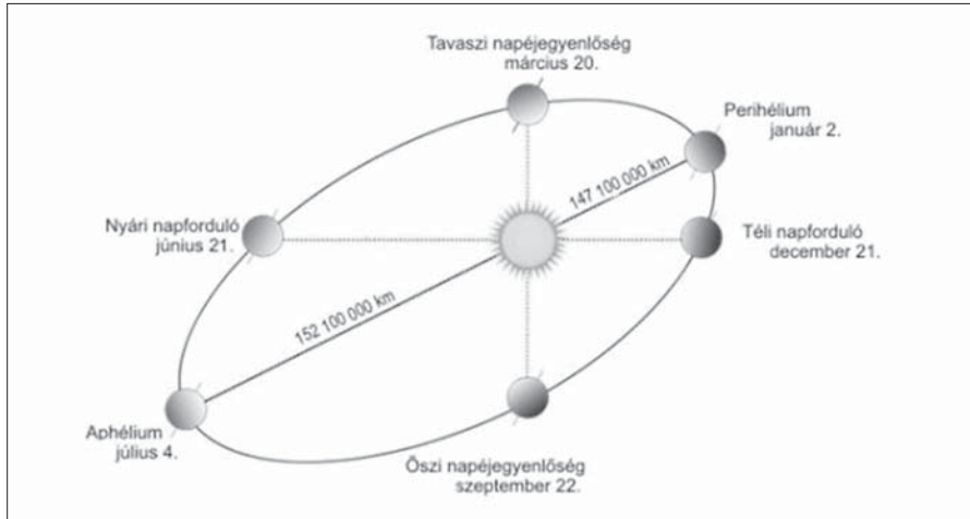
7. ábra. A Föld pályájának sajátosságai és az évszakok váltakozása.
