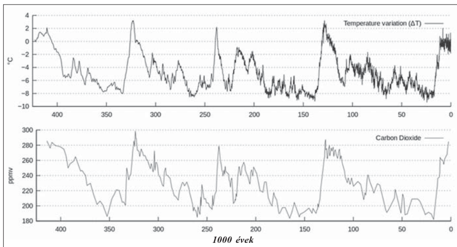
8. ábra. A hőmérséklet (felső adatsor), és a széndioxid koncentráció (alsó adatsor) változása az utóbbi 450.000 évben az antarktisi jégbe csapdázódott légbuborékok analízise alapján.
