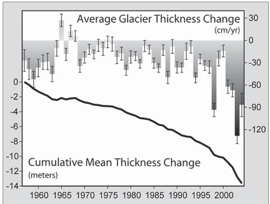
12. ábra. Az átlagos gleccserjég vastagság változása cm/év viszonylatban (éves fluktuáció szórással, jobb oldali skála), valamint összesítve méter/ év dimenzióban kifejezve (folytonos vonal, bal oldali skála).
