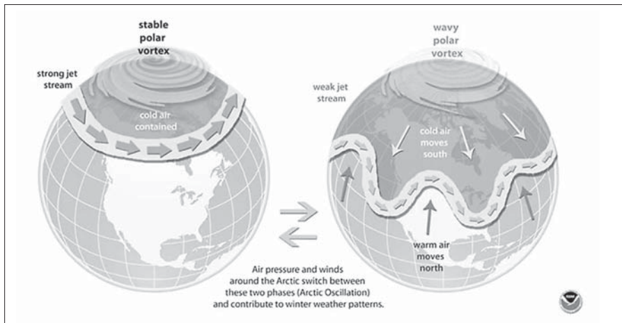
4.A ábra. Az Északi-sarki Örvény stabil és gyenge, hullámzó állapota. Forrás: https://www.noaa.gov/multimedia/infographic/science-behind-polar-vortex
