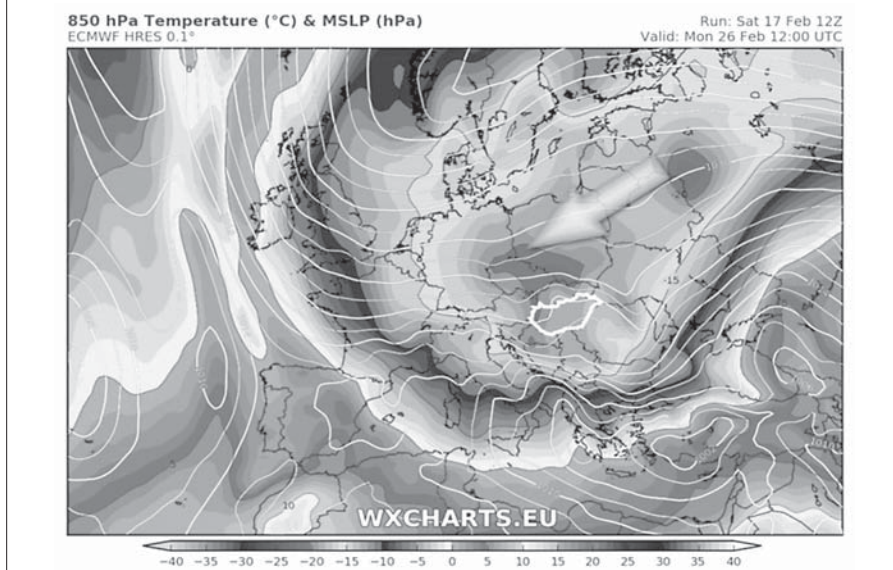
4.B ábra. Hidegbetörés konkrét esetei. Forrás: WXCharts.com Varga Sándor - sandor1 / 2019. november 22. 14:29 https://www.idokep.hu/keptar/album/Id%C5%91j%C3%A1r%C3%A1si%2Bgrafikonok%2C%2Bt%C3%A9rk%C3%A9pek/kep/542816#kep
