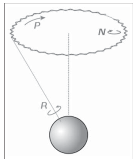
6. ábra. A precesszió és a nutáció hatása a földtengelyre (R – a Föld forgástengelye; P – Precesszió N – Nutáció)
