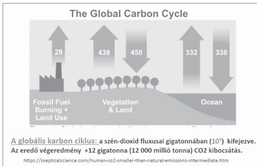
1. ábra. A globális karbon-ciklus szén-dioxid fluxusai gigatonnában (10 9 ) kifejezve. Az első egység a fosszilis üzemanyagok és a földhasználat által kibocsátott szén-dioxid mennyiségét, a középső egység a vegetáció és a szárazföldek, míg a harmadik egység az óceánok, tengerek CO 2 kibocsátását és elnyelését ábrázolják.
