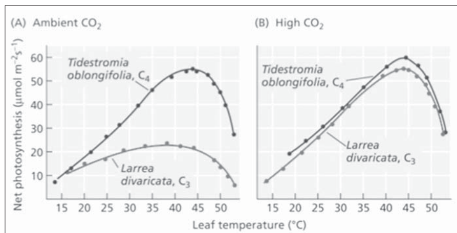
3. ábra. C3-as és C4-es növény fotoszintézis aktivitása a levél hőmérsékletének függvényében alacsony és magas CO 2 koncentráció mellett.
