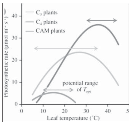
4. ábra. Hőmérsékleti optimumok a C3-as és C4-es növények esetében. A C3-as optimális tartomány 15-25 °C fok között, a C4-es 30-40 °C fok között van (a „CAM” növények – alsó görbe – esetünkben nem fontosak).
