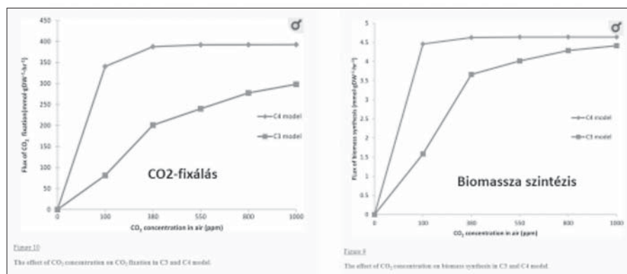
2. ábra. A C3-as fotoszintézis a CO 2 koncentráció emelkedésével hatékonyabb lesz.
